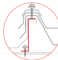
FRP/ACERO (Gancho Z)
