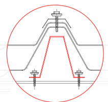
Fijación intermedia
